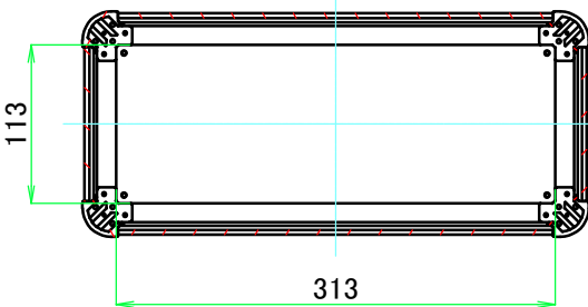
C-C ( 1 : 6 )
