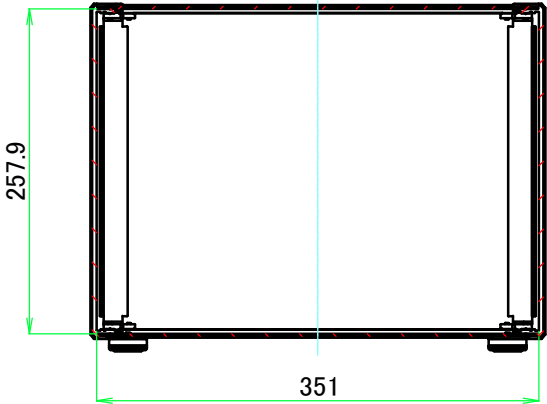
A-A ( 1 : 6 )
