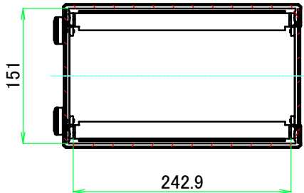
B-B ( 1 : 6 )
